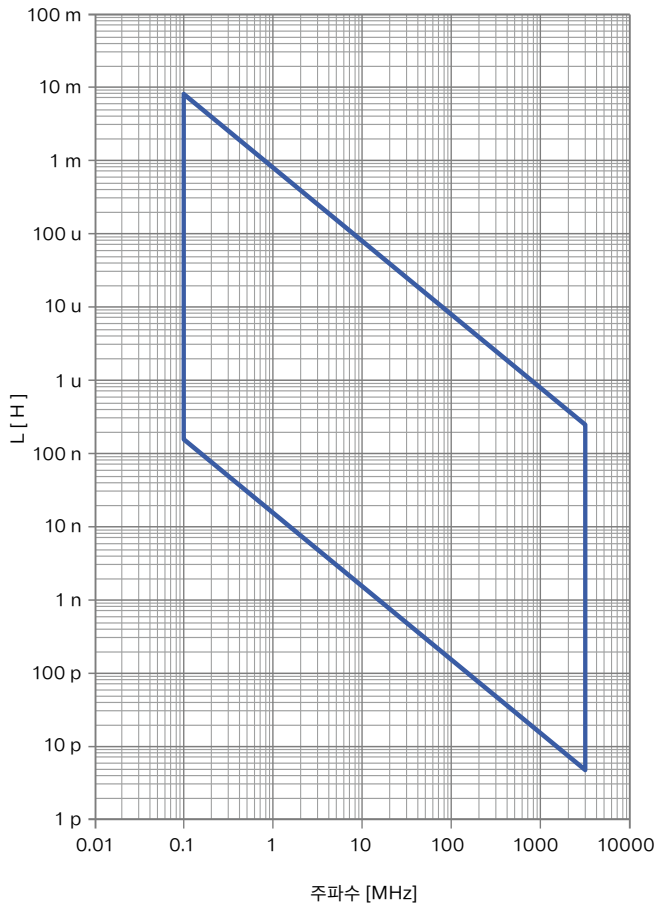
L 측정가능범위
