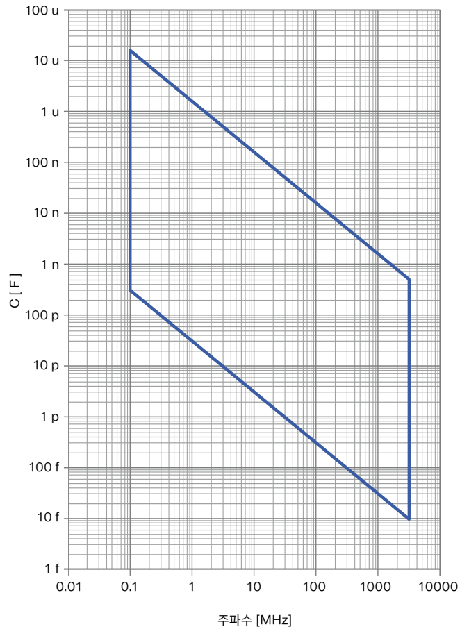
C 측정가능범위
